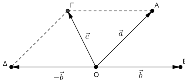
Σχήμα 1: Αφαίρεση διανυσμάτων
